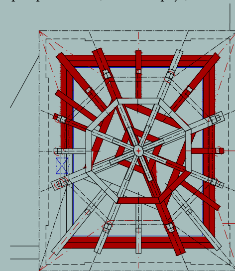
Rozsah poškození východní věže.
